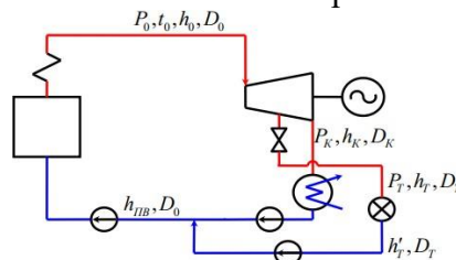
Рисунок 13.1 – Схема паротурбинной установки с отпуском тепла потребителю
