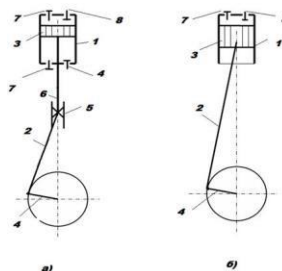
Рисунок 10.7– Конструкции механизма движения компрессора
