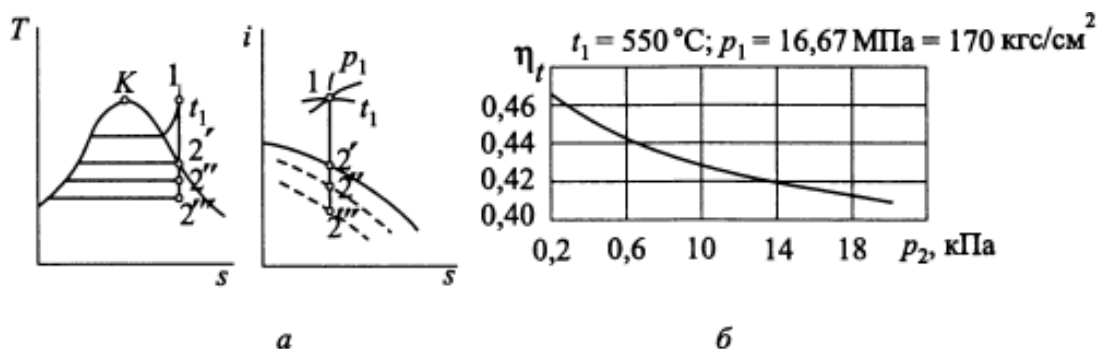
Рисунок 5.4. Влияние понижения давления в конденсаторе на влажность пара в конце расширения (а) и экономичность цикла Ренкина (б)
