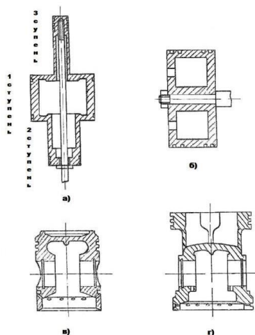
Рисунок 10.14 – Поршни компрессоров
