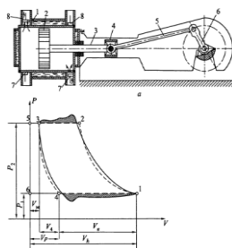
а - схема: 1- цилиндр; 2 - поршень; 3 - шток; 4 - крэйцкопф; 5 - шатун; 6 - кривошип; 7 и 8 - всасывающий и нагнетательный клапаны; б - индикаторная диаграмма (цифры на диаграмме соответствуют точкам процесса)
