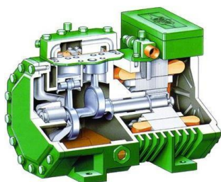
Рисунок 10.11 – Прямоточный компрессор
