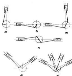
Рисунок 10.8 – Расположение осей цилиндров компрессоров
