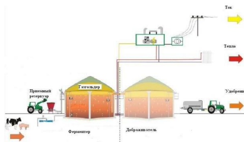
Рисунок 3.13 - Схема биогазового энергетического комплекса
