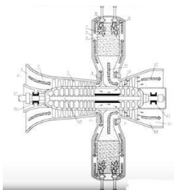
Рисунок 9.8 – Устройство современных газотурбинных установок
