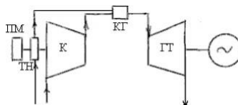
Рисунок 9.5 - Простейшая схема газотурбинной установки
