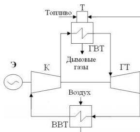
Рисунок 9.11 - Замкнутая схема работы ГТУ:
