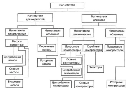
Рисунок 10.1 - Классификация нагнетателей
