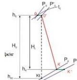
Рисунок 13.4 – Процесс расширения пара в турбине без отборов
