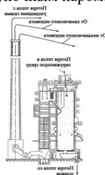
Рисунок 8.6 - Основные потери теплоты
