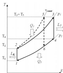
Рисунок 9.9 - Идеальный цикл Брайтона: 1–2–3–4–1 — подвод теплоты при p=\text{const} ; 1–2–5–6–1 — подвод теплоты при v=\text{const}
