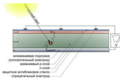
Рисунок 3.5 - Простейшая конструкция солнечного элемента (СЭ)
