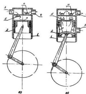
Рисунок 10.9 – Схема прямоточного (а) и непрямоточного (б) компрессор
