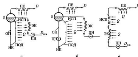
Рисунок 8.2 - Схемы генерации пара в паровых котлах: а - естественная циркуляция; б - многократная принудительная циркуляция; в - прямоточная схема; Б - барабан; ИСП - испарительные поверхности; ПЕ - пароперегреватель; ЭК -
