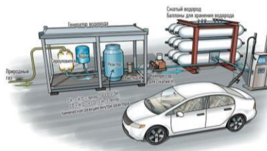
Рисунок 7.13 - Для получения водорода применяется электролиз, после его генерации водород сжимается или сжижается и хранится для последующего его использования в генераторах или топливных элементах. Изображение предоставлено компанией Affiliated Engineers
