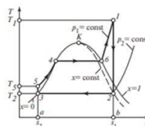
Рисунок 9.4 – Цикл Ренкина в T-S диаграмме
