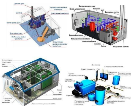
Рисунок 8.5 - Примеры компоновки некоторых котельных и их оборудования
