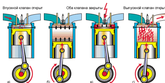
Рисунок 12.6 - Рабочий цикл четырехтактного карбюраторного двигателя: а) впуск; б) сжатие; в) рабочий ход; г) выпуск
