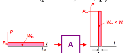
Рисунок 7.3 – Применение аккумулятора энергии (А) для получения импульса энергии повышенной мощности
