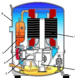
1 – электродвигатель , 2 – коленчатый вал , 3 – шатунно-поршневая группа, 4 – блок цилиндров, 5 – глушитель шума , 6 – кожух.
