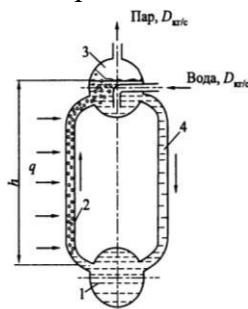
Рисунок 8.3 - Схема естественной циркуляции воды в котле: 1 - нижний коллектор; 2 - левая труба (экран); 3 - барабан котла; 4 - правая труба
