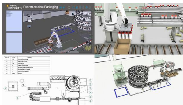
Рисунок 15.5 - Проектирование роботизированной линии фармацевтического производства
