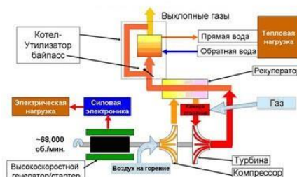
Рисунок 15.2 – Общая схема микротурбинной электростанции
