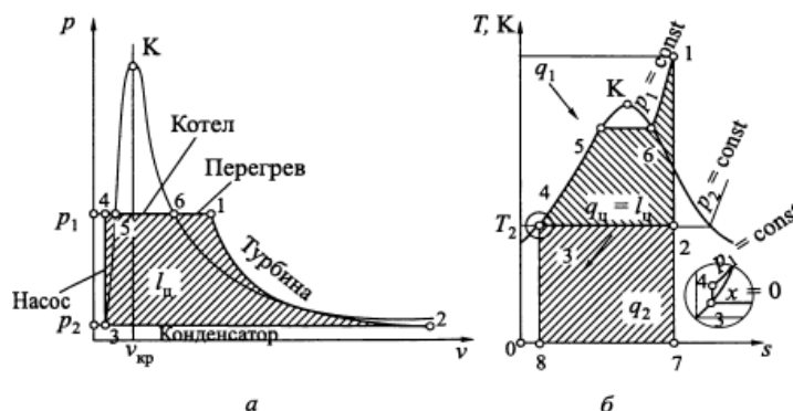
Рисунок 5.2 - Цикл Ренкина на перегретом паре в p, v а- T, s б-диаграммах
