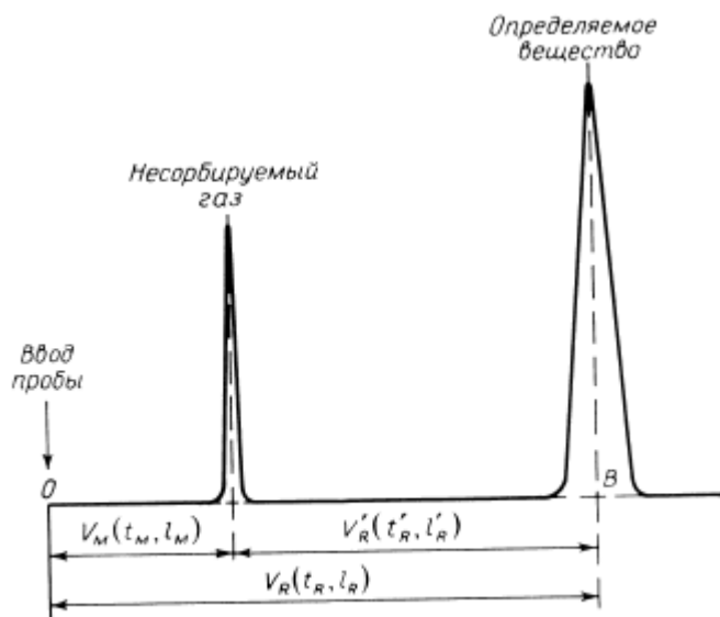
Рис.1.Общий вид хроматограммы
