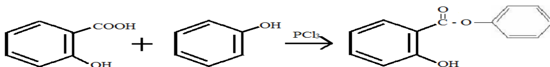
Фенилсалицилат (салол)
