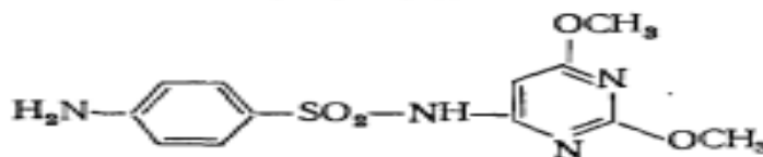
Сульфадиметоксин
