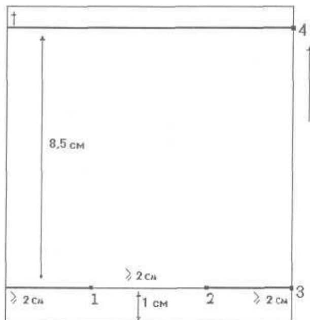
Рис. 3. Разметка пластины:
