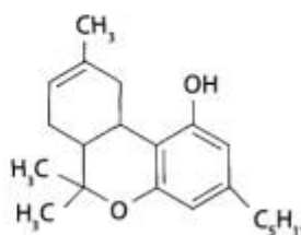
\Delta^8 -тетрагидроканнабиол ( \Delta^8 -ТГК)
