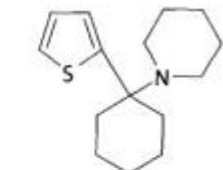
тиеноциклидин 1-(1-(2-тиенил)-цикло- гексил)-пиперидин
