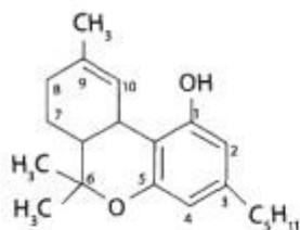
\Delta^9 -тетрагидроканнабиол \Delta^9 -ТГК
