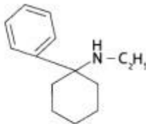
этициклидин N-(1-фенилциклогексил) этиламин
