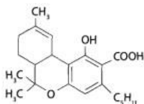
\Delta^9 -тетрагидроканнабиол-2-карбоновая кислота ( \Delta^9 -ТГК-кислота)
