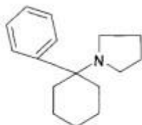
ролициклин 1-(1-фенилциклогексил) пирролидин
