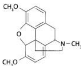
тебаин
