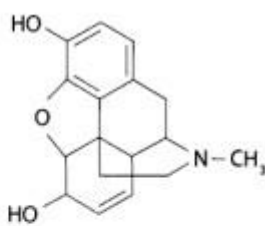
морфин
