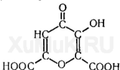
Меконовая кислота
