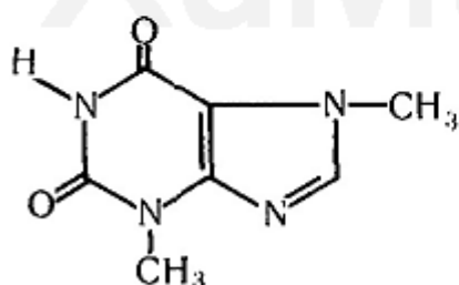
Теобромин (3,7-диметилксантин)
