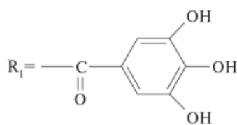
Галловая кислота
