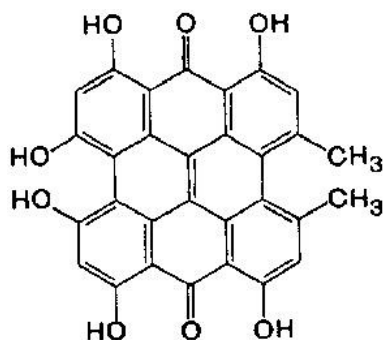
Гиперичин
