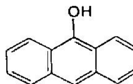
Антранол
