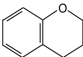
Хроман
