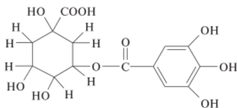
Теогаллин (депсид)
