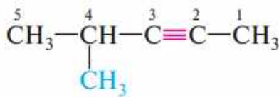
4-метил-2-пентин
